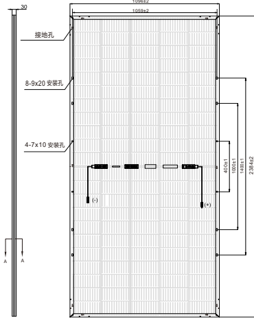
产品图示 单位: mm
